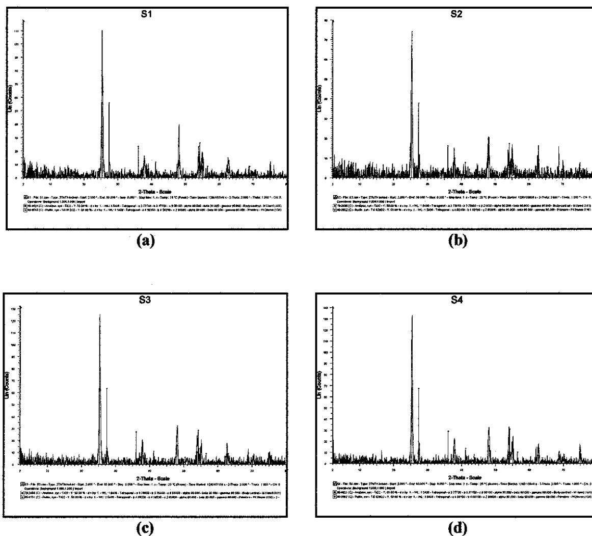
Figure 4.7: XRD diffractograms for Fe/TiO 2 (a) 0.1Fe_5 (b) 0.5Fe_5 (c) 1.0Fe_5 and (d) 1.0Fe_4
